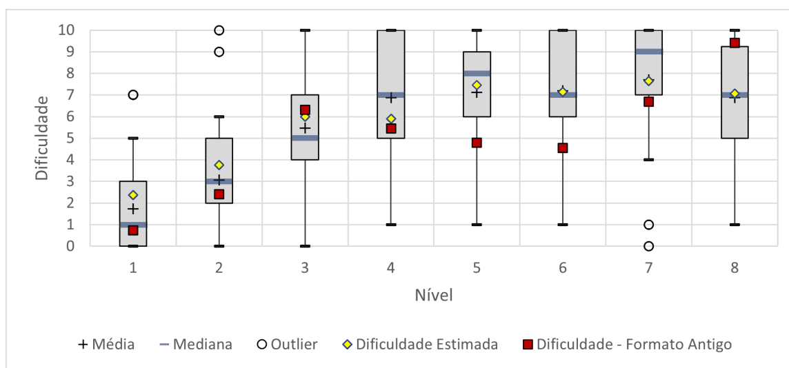
Figura 6.5: Diagrama de caixa com as médias das dificuldades experienciadas pelos jogadores, medidas por meio do questionário, e os valores estimados por algoritmos na primeira bateria de testes. A estimação de dificuldade pelo método atualizado está em amarelo e a estimação pelo método anterior está normalizada e em vermelho.
