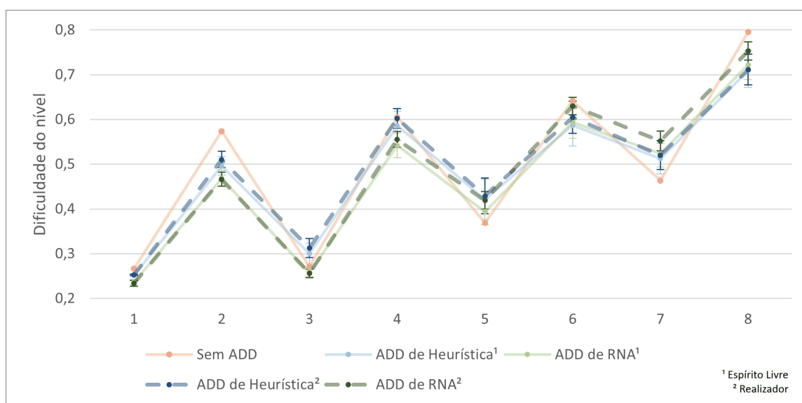
Figura 6.40: Média e desvio padrão de cada nível ao adaptar para os participantes da terceira bateria de testes, divididos por modelo de ADD pela cor e pelo perfil de jogador predominante entre Espírito Livre e Realizador pelo tracejado das linhas.
